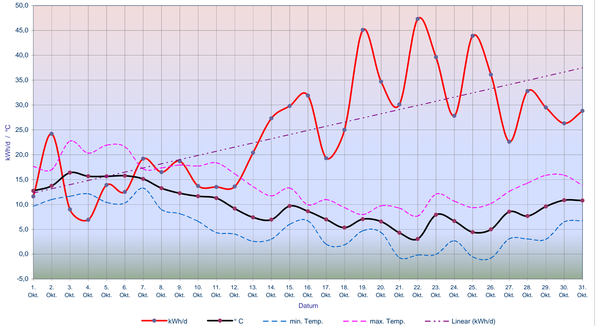
Tages-Energieverbrauch (kWh/d) bezogen auf 156,7 m 2 Wohnfläche Solarthermie: 15,2 m 2 mit Hz.-Unterstützung (Süddach 38° DN)
