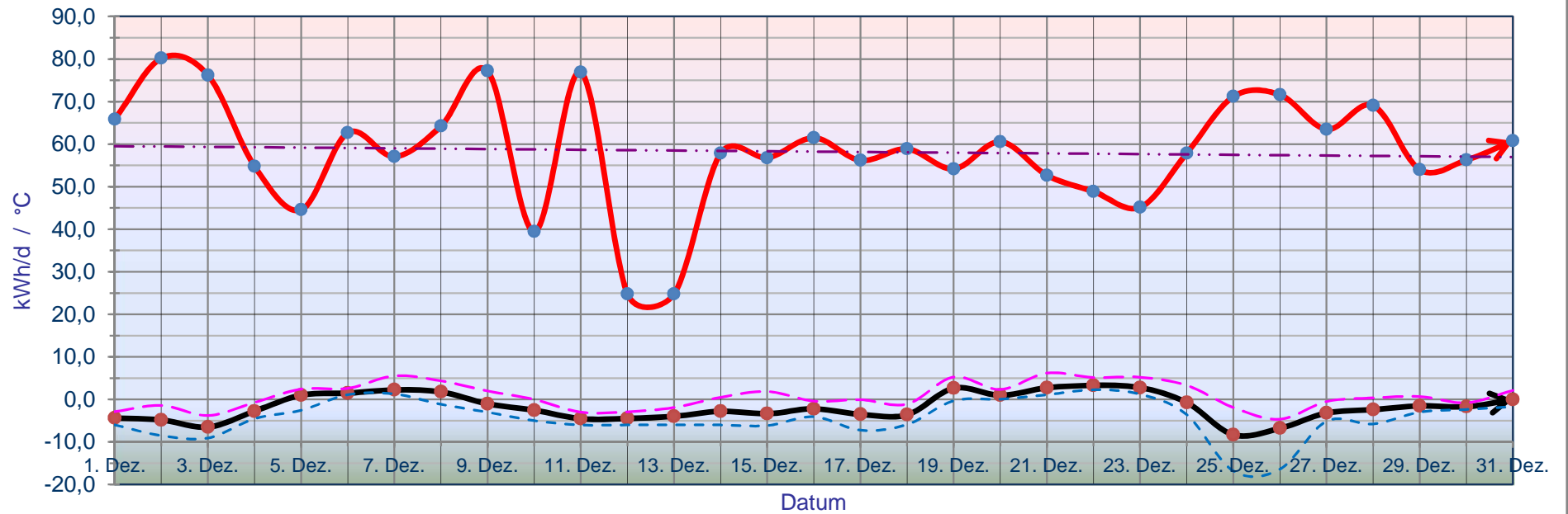
Tages-Energieverbrauch (kWh/d) bezogen auf 156,7 m 2 Wohnfläche Solarthermie: 15,2 m 2 mit Hz.-Unterstützung (Süddach 38° DN) Dezember 2010
